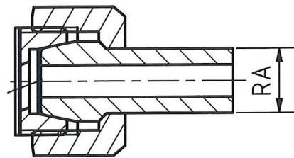
Verschraubungsart AV2 screw option AV2
