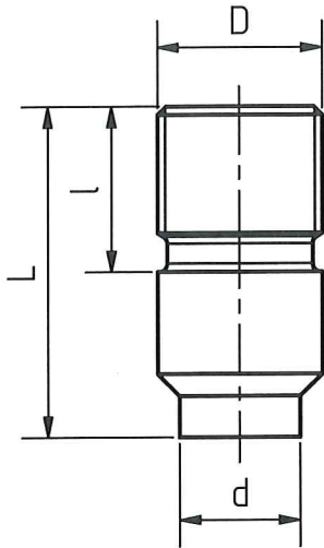
Schweißstutzen
