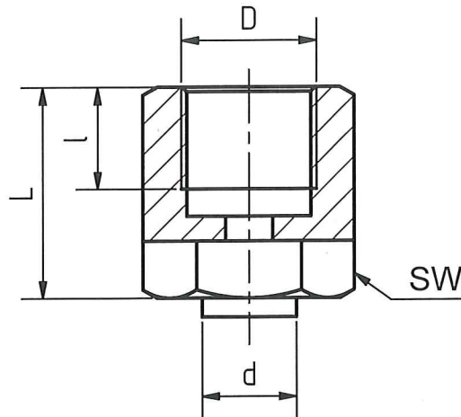
Schweißmuffe
